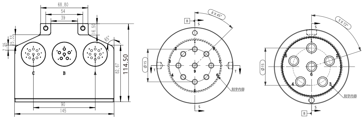
HP-K24外形尺寸图:
