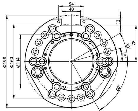
SQ-200T外形尺寸图:
