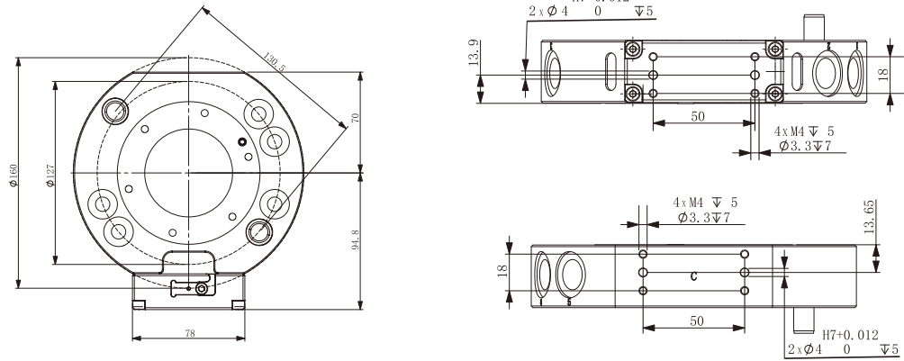
SQ-100T外形尺寸图:
