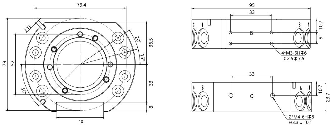
SQ-25T外形尺寸图:
