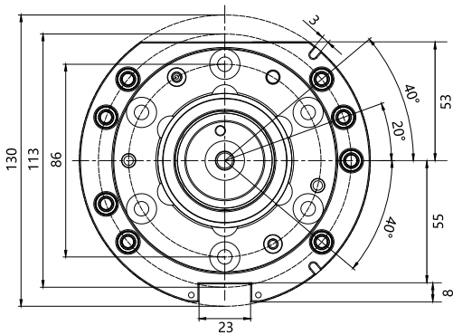
HQ-75外形尺寸图:
