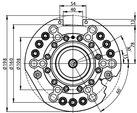
HQ-200外形尺寸图:
