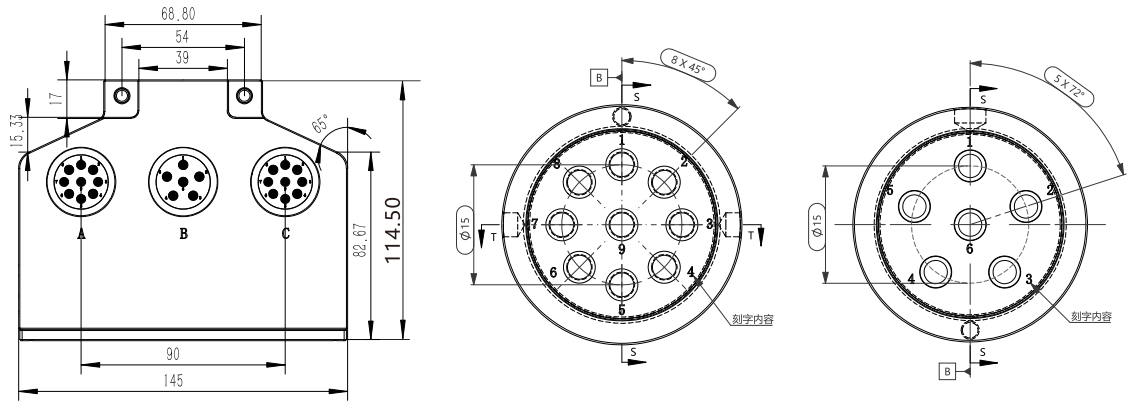
HT-K24外形尺寸图:
