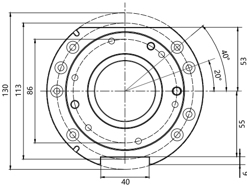
SQ-75T外形尺寸图:
