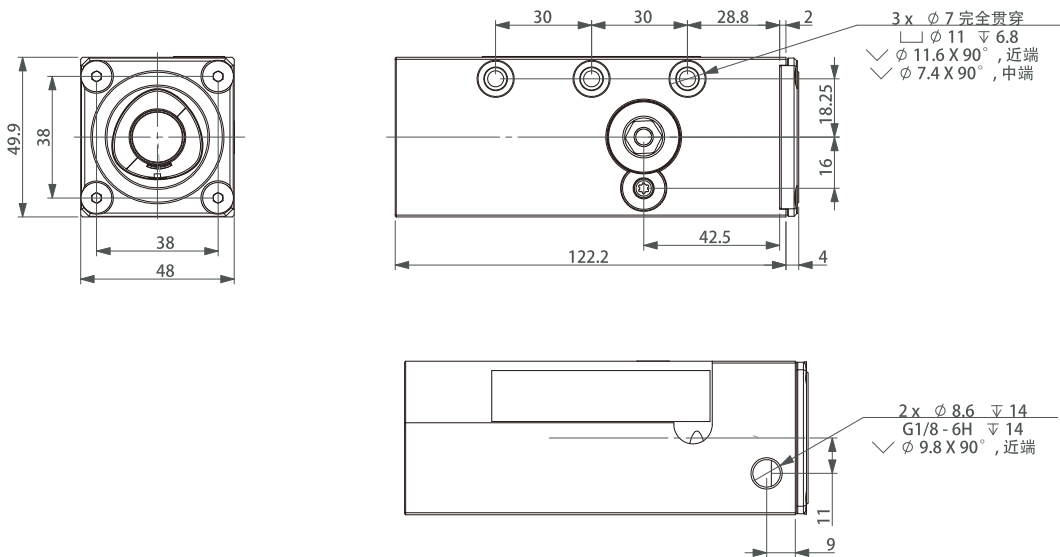
外形尺寸表
